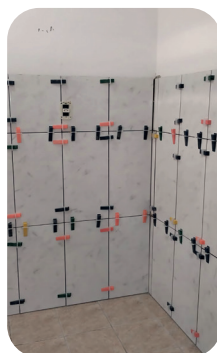
REFORMA APARTAMENTOS
